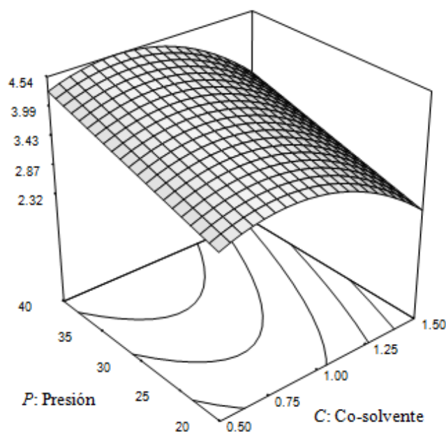
Figura 4.3 Superficie de respuesta para actividad antiinflamatoria ( Y_3 , IC_{50} mg/ mL), en función de la presión ( P , MPa) y uso de co-solvente ( C , %p/p).
