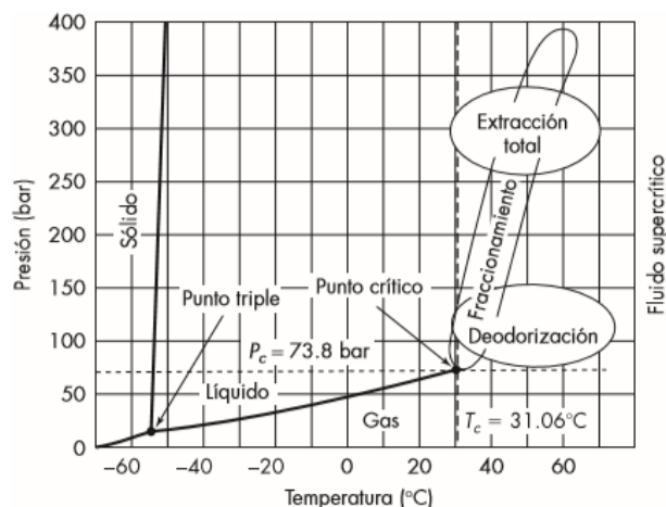
Figura 2.1 Diagrama de fases para el dióxido de carbono, que ilustra regiones útiles para las aplicaciones en el procesamiento de alimentos (McCabe et al. , 2007).
