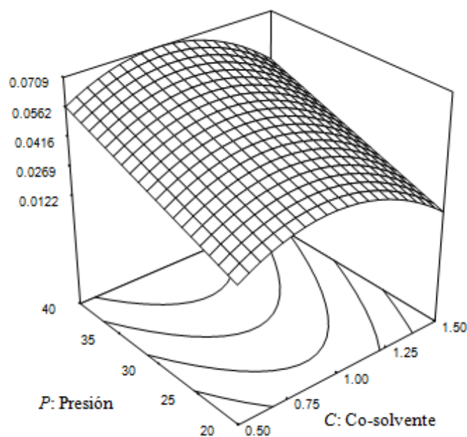
Figura 4.2 Superficie de respuesta para la extracción de antioxidantes ( Y_2 , mmol TE/ kg SS), en función de la presión ( P , MPa) y uso de co-solvente ( C , %p/p).
