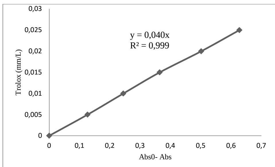
Figura B-1. Curva de calibración para el ensayo del radical DPPH.
