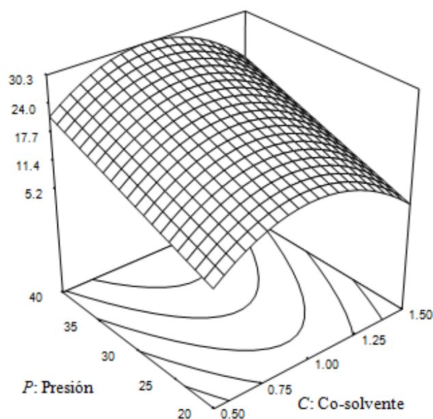
Figura 4.1 Superficie de respuesta para rendimiento de extracción ( Y_1 , g/ kg SS), en función de la presión ( P , MPa) y uso de co-solvente ( C , %p/p).
